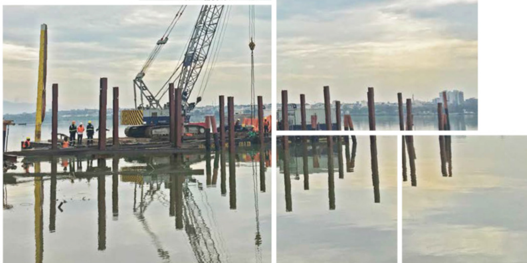
Jetty Construction
